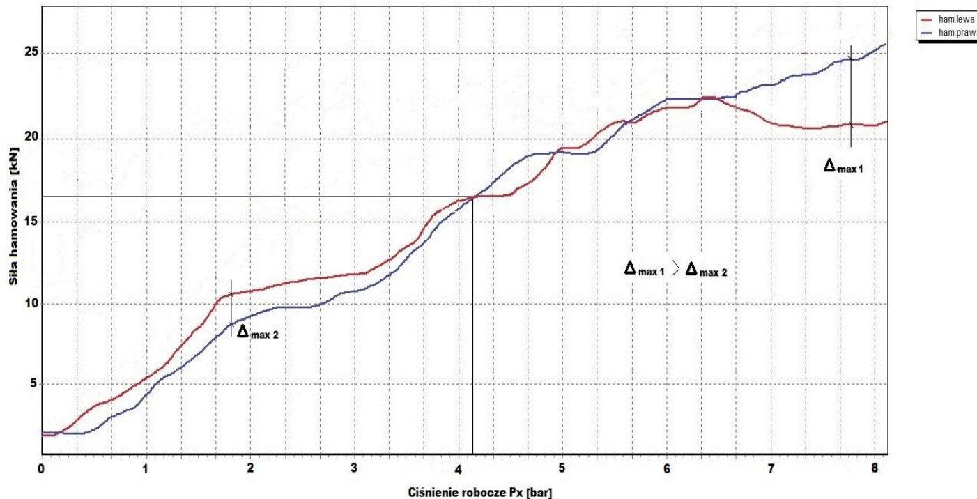
Siła hamowania od ciśnienia roboczego P_x OŚ 2 HR
